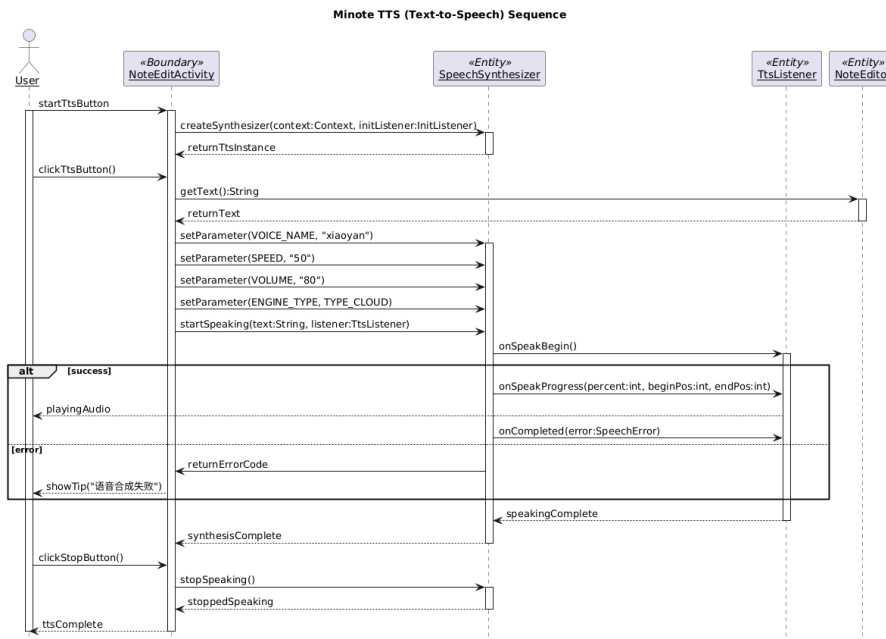
图 51: 朗读功能的时序图
