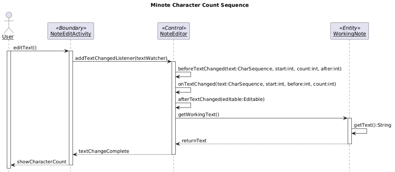
图 43: 统计字符个数的时序图
