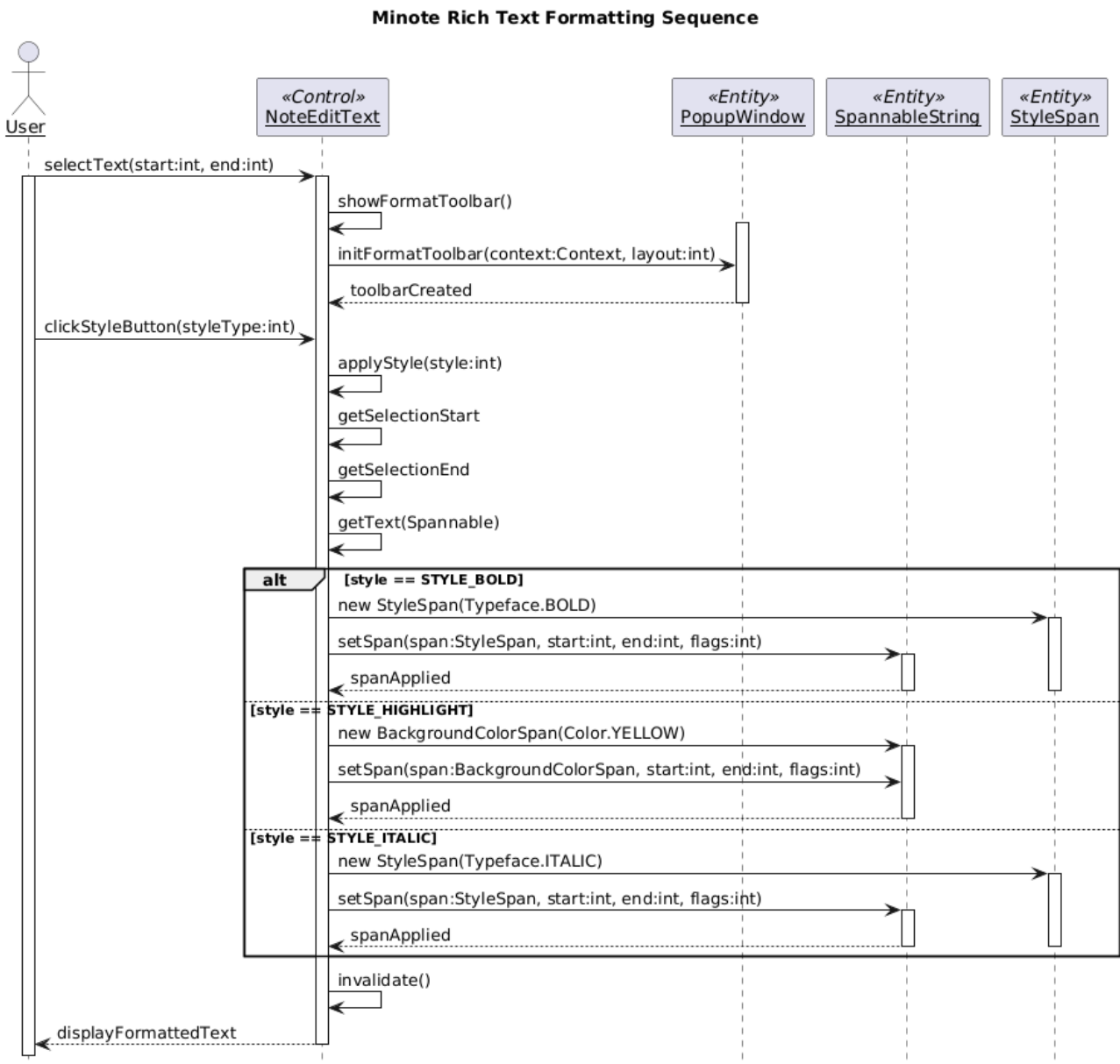
图 49: 富文本功能的时序图
