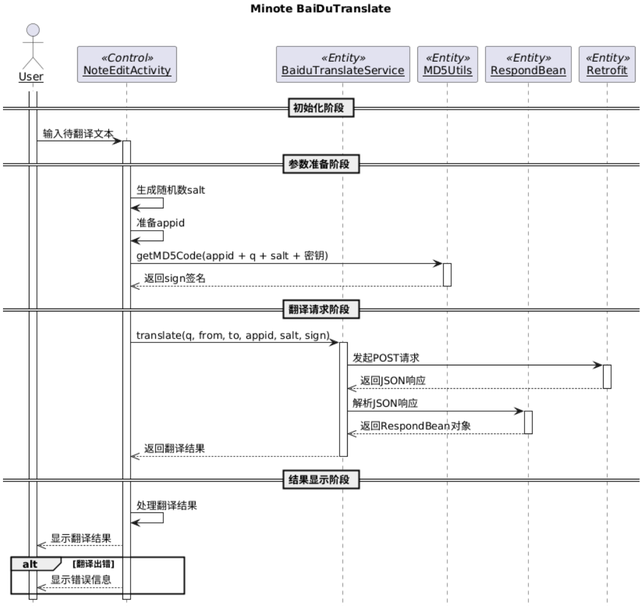
图 39: 翻译功能的时序图
