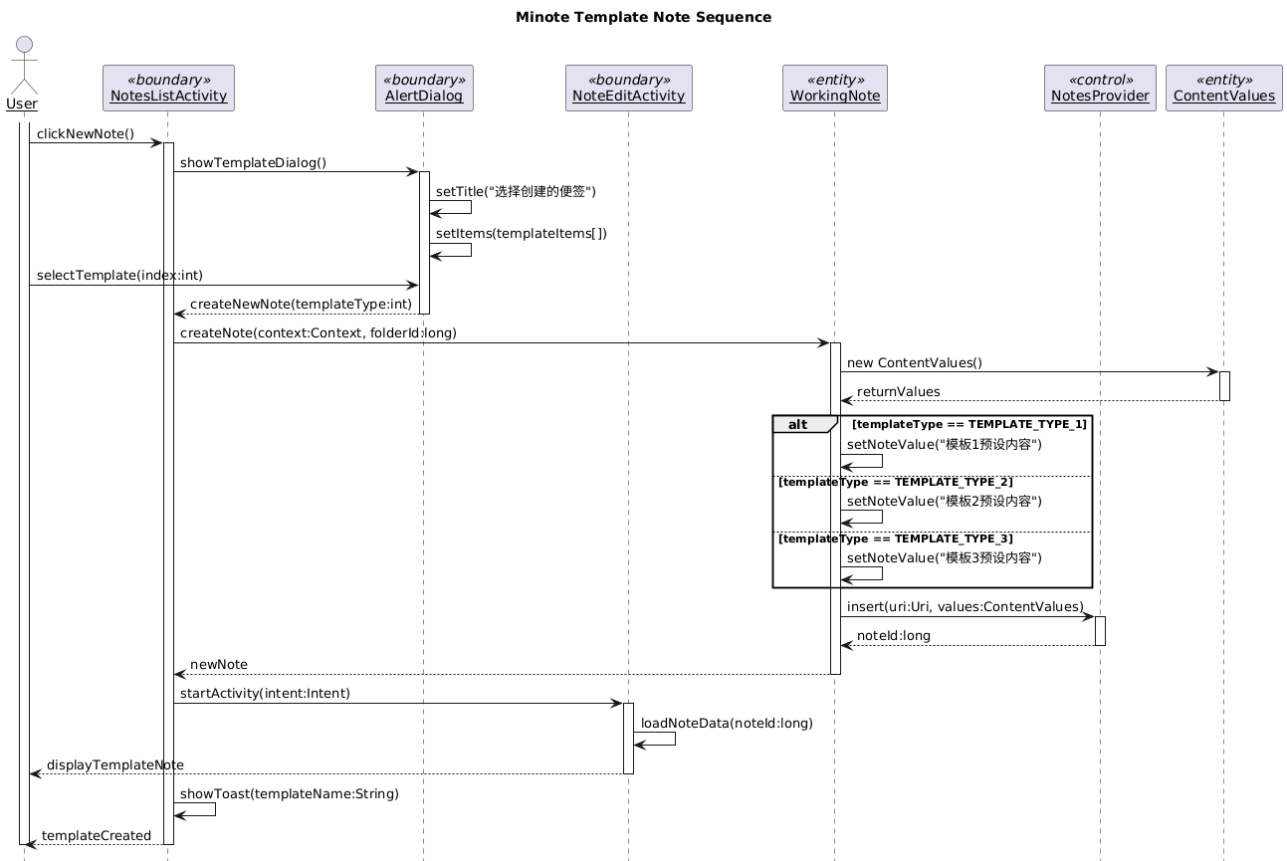
图 62: 模板便签的时序图
