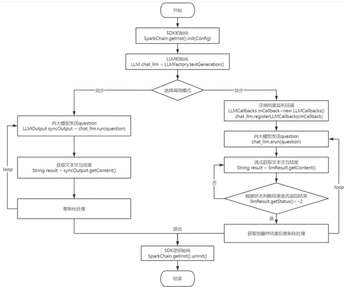
图 71: 对话式大模型的流程图
