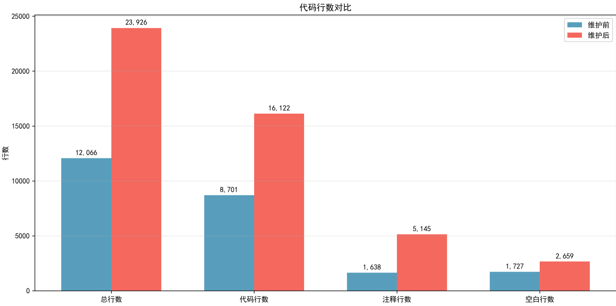
图 22: 维护前后代码数量对比——柱状图
