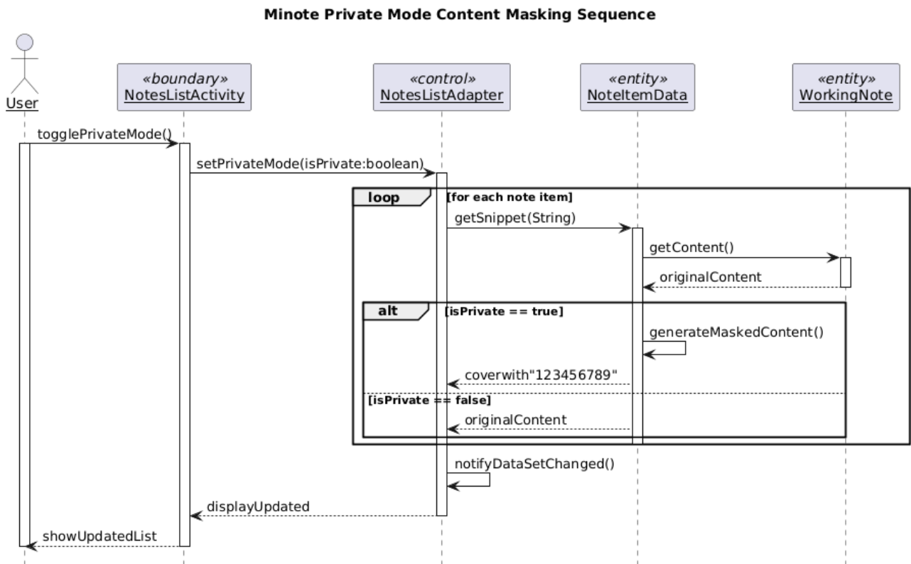
图 54: 私密模式的时序图
