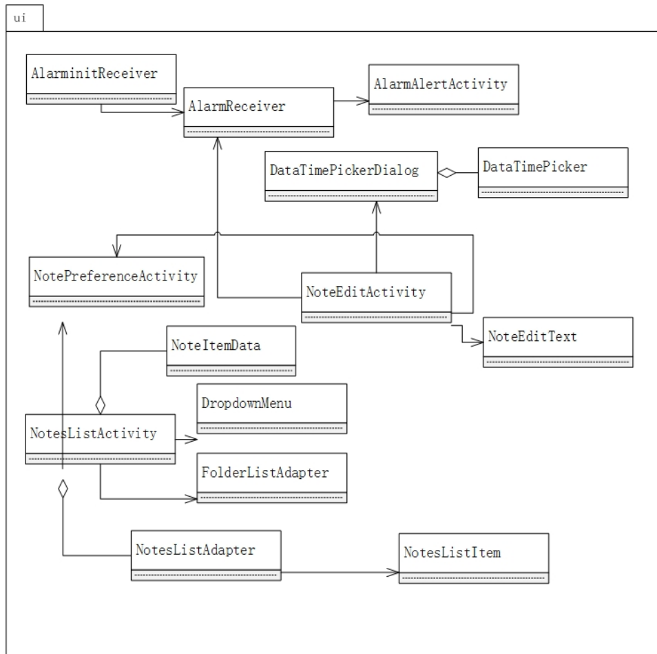
图 8: ui子系统 中的类图
