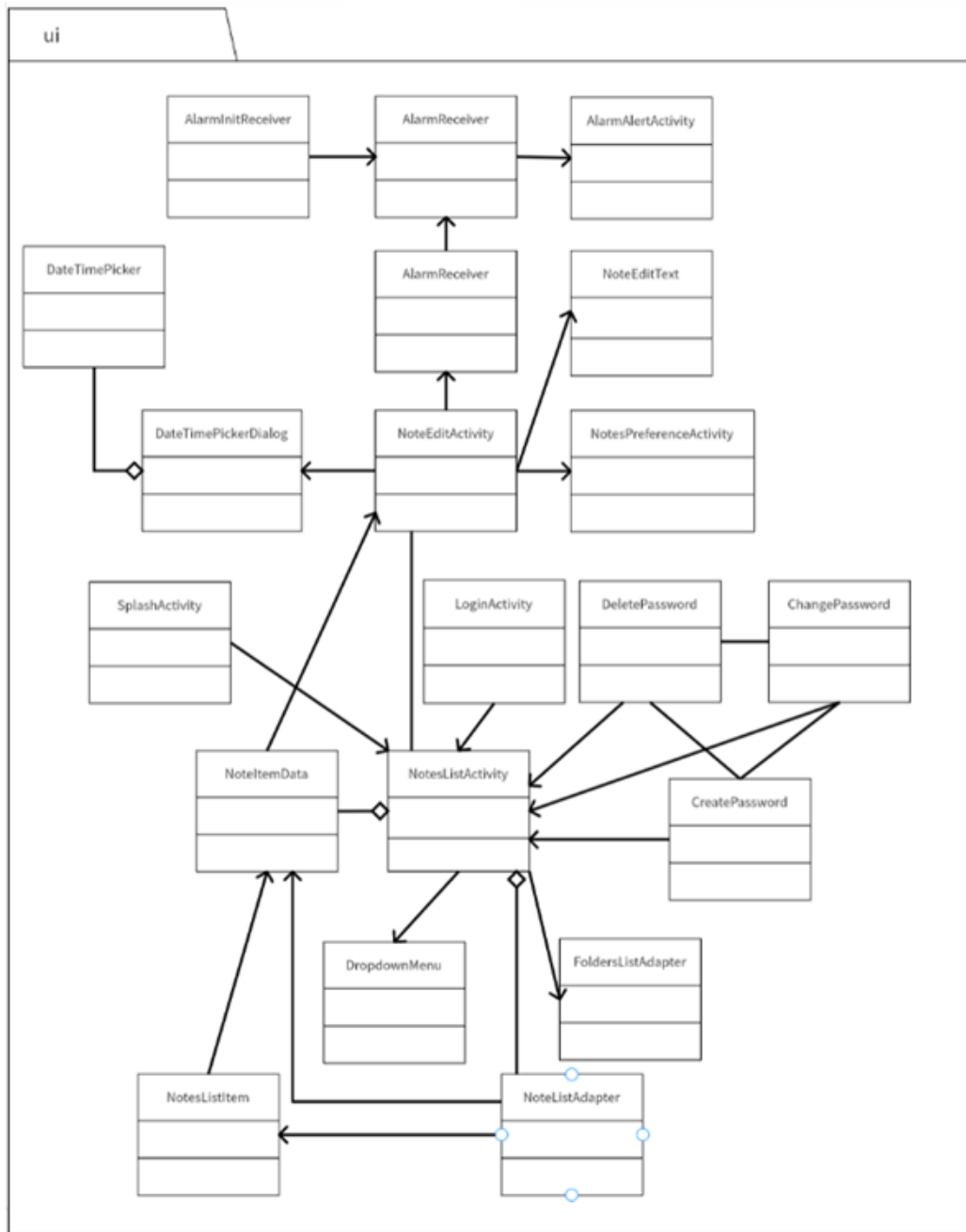
图 11: 维护后ui包内的类图
