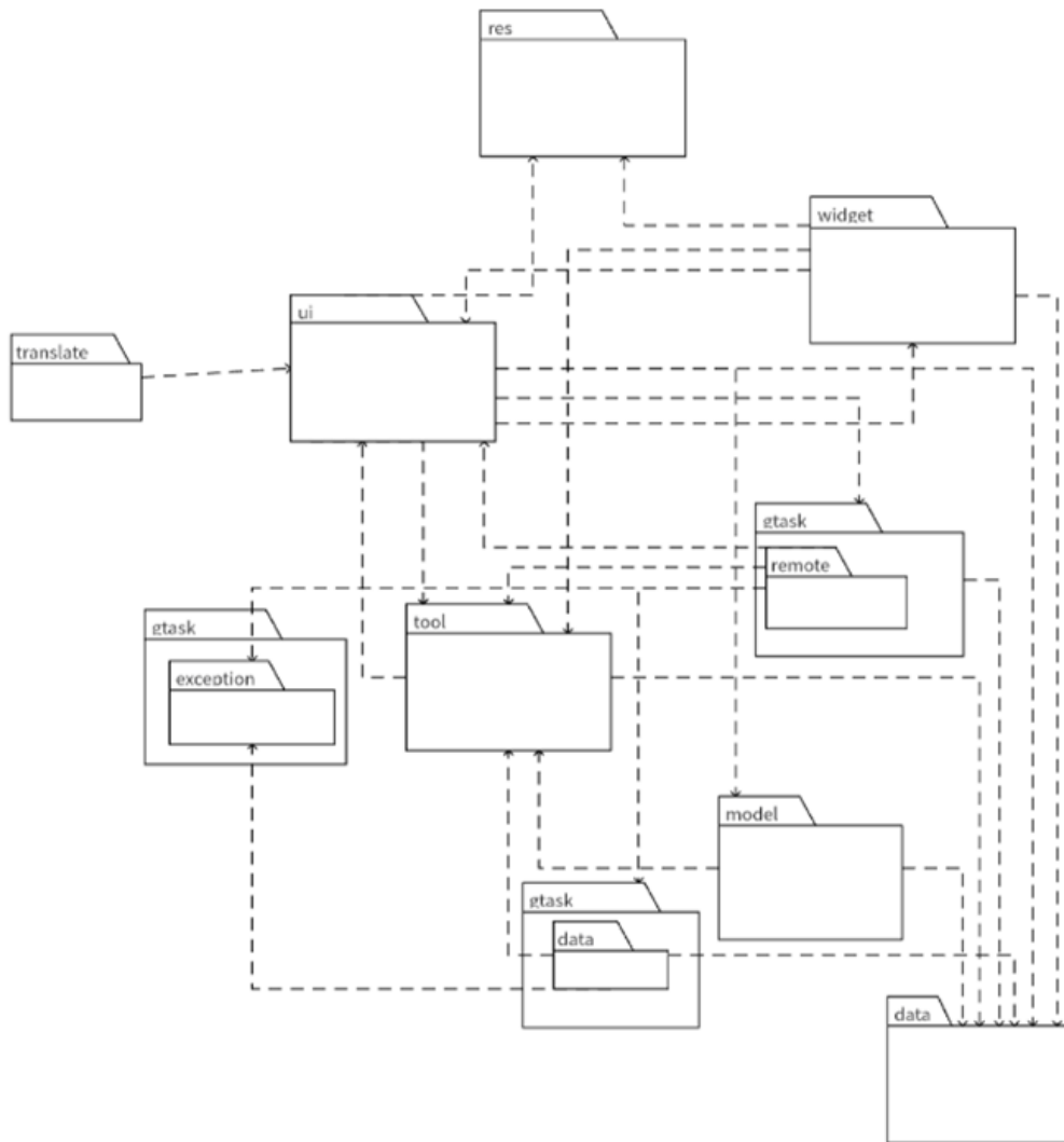
图 10: 维护后的小米便签包图
