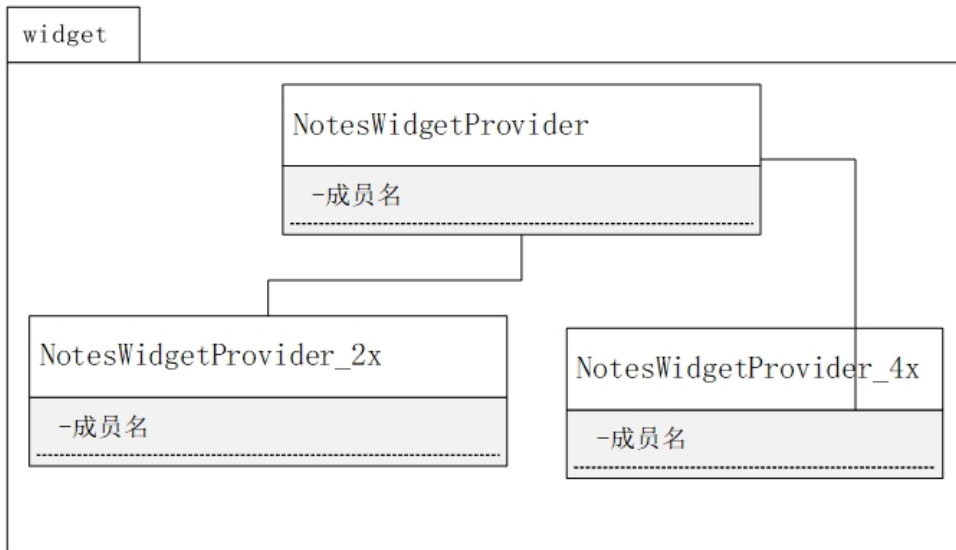
图 6: widget 子系统 中的类图
