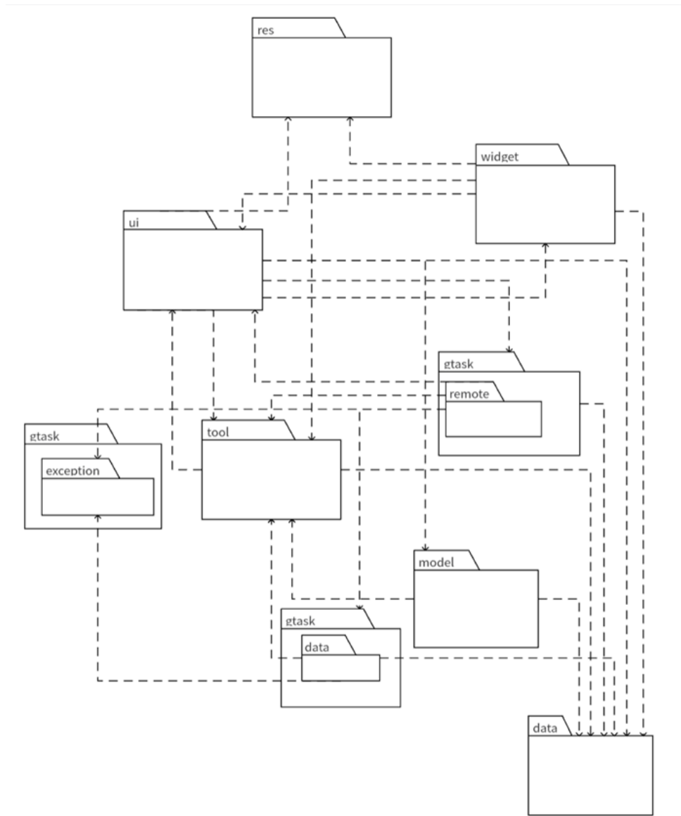
图 3: 小米便签的包间关系图
