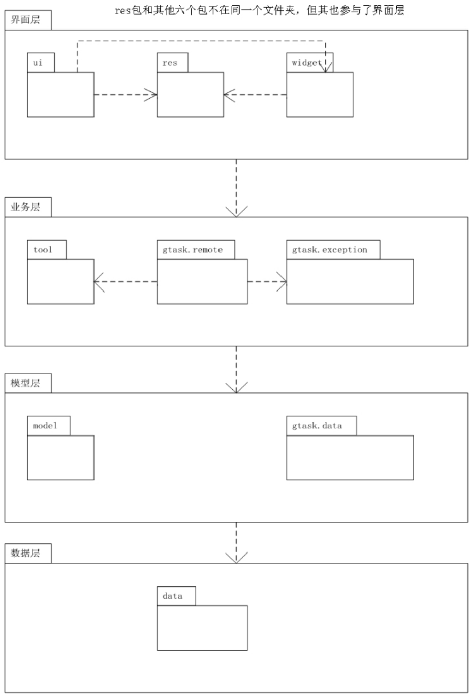
图 2: 小米便签的软件架构图
