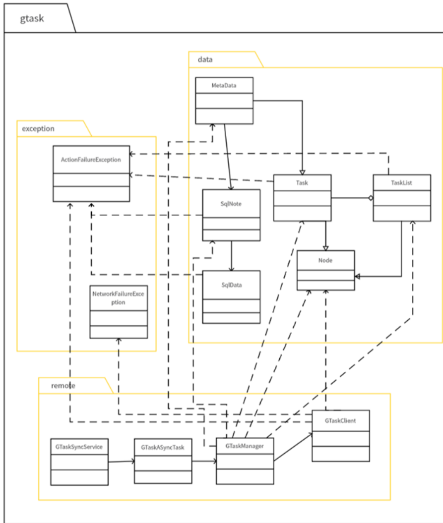
图 9: Gtask子系统类中的类图
