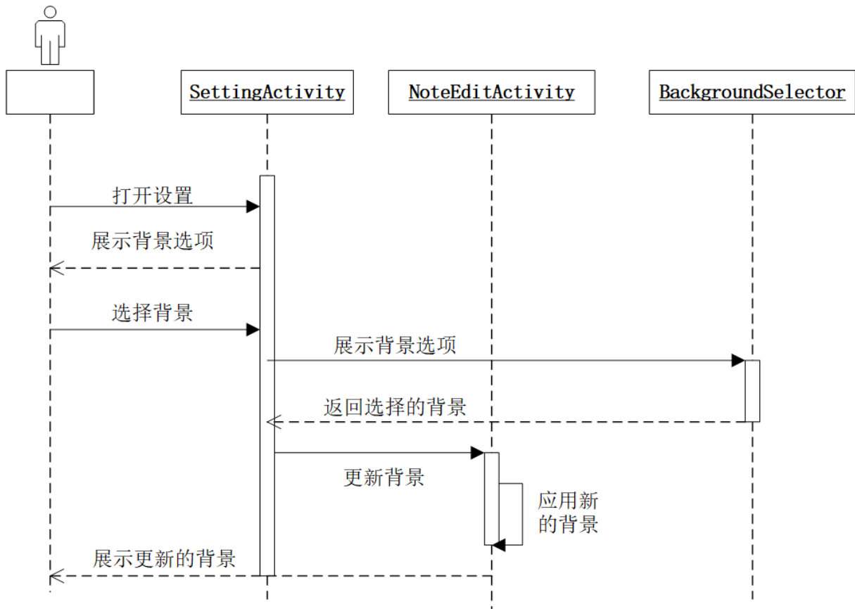
图 13: 设置界面背景的时序图
