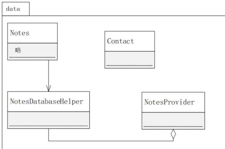
图 4: data 子系统 中的类图
