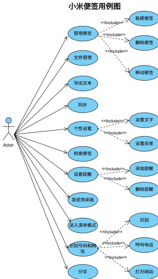
图 1: 小米便签的软件需求用例图
